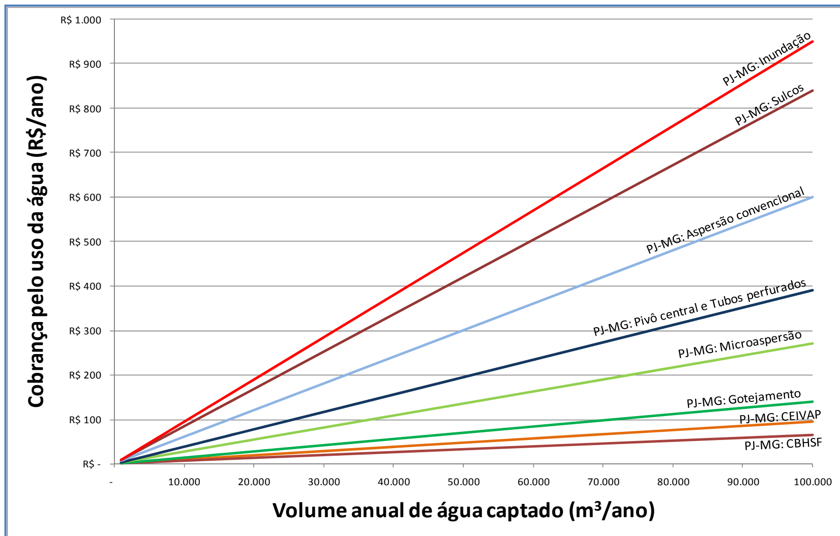
Figura 1 – Cobrança pelo uso da água para irrigação de acordo com diversos mecanismos e técnicas
